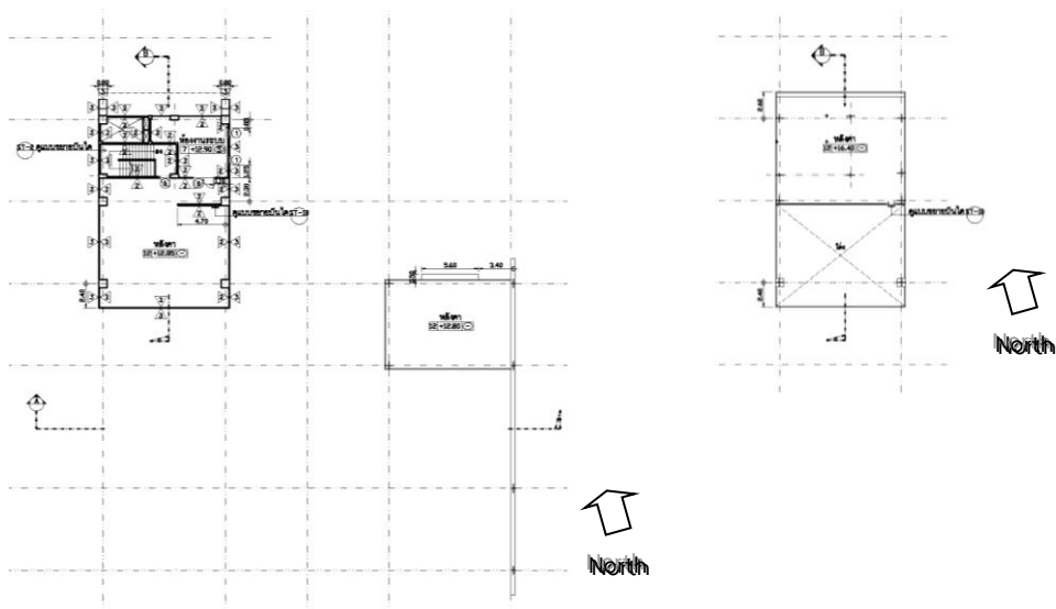
ภาพที่ 5 แสดงแปลนพื้นที่ชั้นหลังคา
