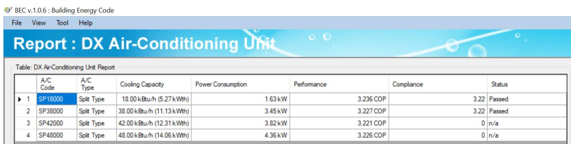
ภาพที่ 9 แสดงค่า COP ของเครื่องปรับอากาศแต่ละขนาด
