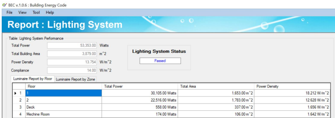
ภาพที่ 8 แสดงค่าการใช้พลังงานไฟฟ้าของระบบไฟฟ้าแสงสว่างแยกตามชั้น
